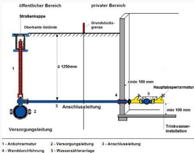
TW-ANSCHLUSS MIT UNTERKELLERUNG DES GEBÄUDES
