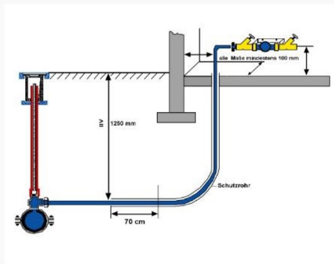
TW-ANSCHLUSS OHNE UNTERKELLERUNG DES GEBÄUDES - IM SCHUTZROHR
